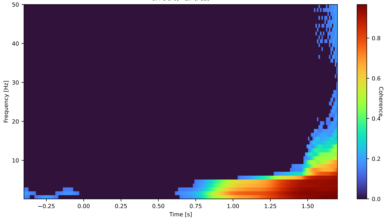
dPFC (F6) - LIP (P13)
